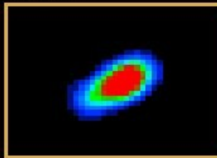
Far-Infrared : IRAS
