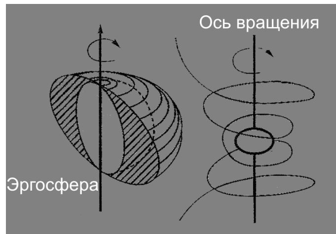
Рис. 12. Структура вращающейся черной дыры. Горизонт событий помещен внутри эргосферы, в которой имеется вихревое гравитационное поле. Луч света, проходящий через эргосферу, завихряется.
