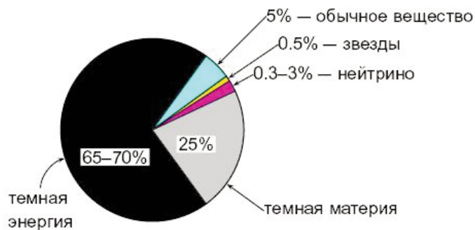
Рис. 1. Состав «энергетической смеси» Вселенной.
