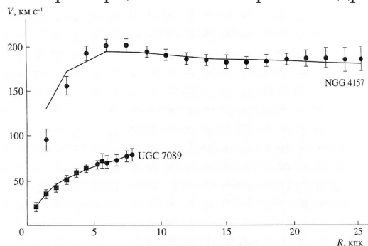
Рис. 5. Распределение линейной скорости вращения галактик по радиусу. На периферии скорость вращения становится почти постоянной и равна большой величине, порядка нескольких сотен км/с. Это свидетельствует о наличии темной материи.
