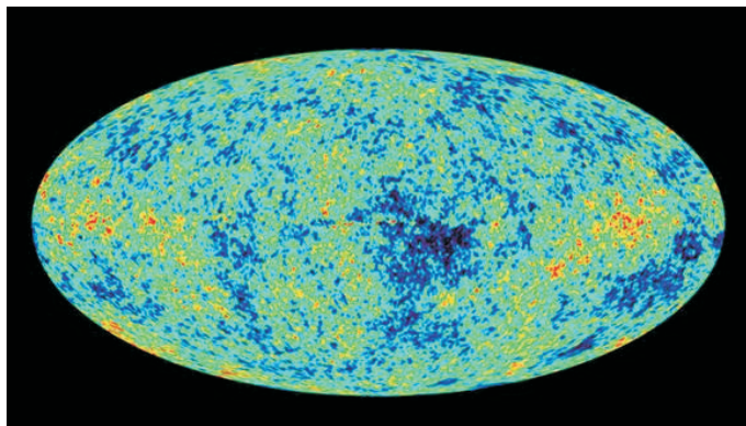
Рис. 10. Распределение флуктуаций интенсивности реликтового излучения по небу. © NASA / WMAP Science Team
