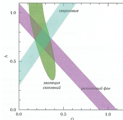
Рис. 11. Зависимости между плотностью темной энергии и плотностью всех остальных видов материи во Вселенной, полученные по наблюдательным данным разных типов. Все три зависимости пересекаются в одной области.
