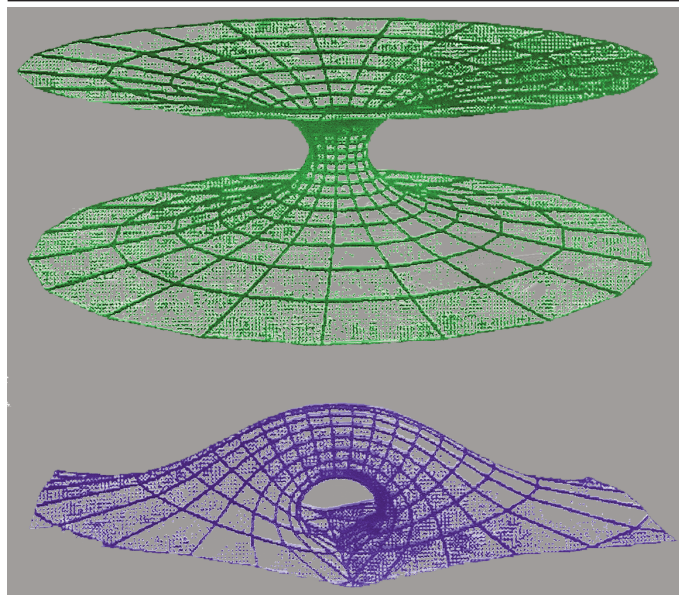
Рис. 14. Двумерное изображение кротовой норы, соединяющей две вселенные (вверху) и две области одной вселенной (внизу).
